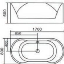
SWP-BT-087 Size : 1700 x 800 x 600mm
