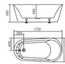
SWP-BT-109 Size : 1700 x 810 x 680mm
