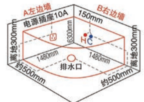
SWP-JC-7113 Size : 1480 x 1480 x 630mm
